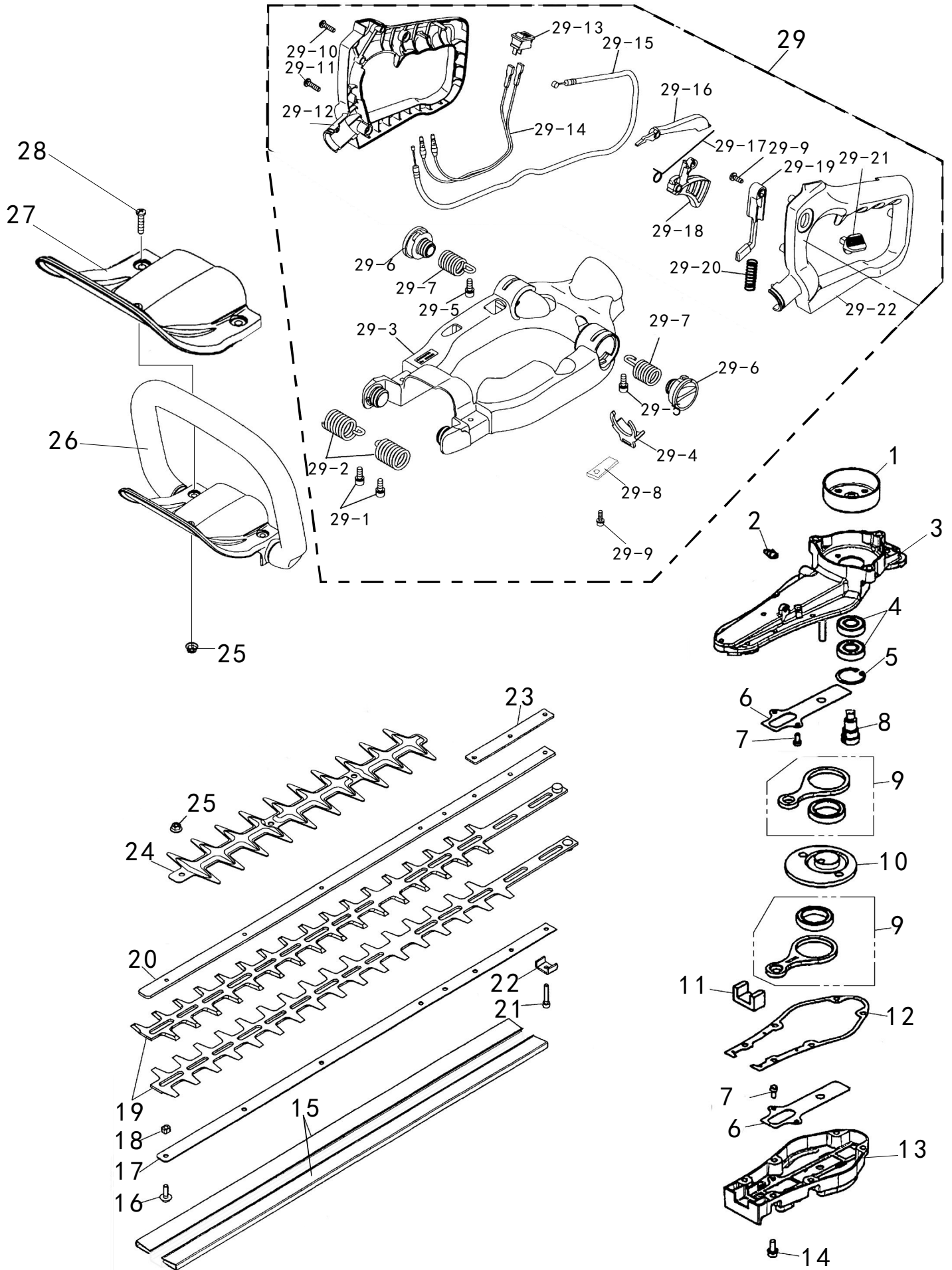
绿篱剪工作头爆炸图
